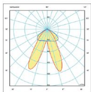
6xDA25°(DA)
